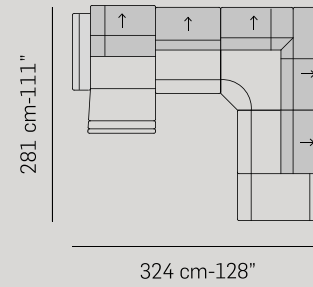
PISA p.118-119
