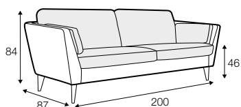
2,5 seater
