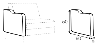
armrest D
