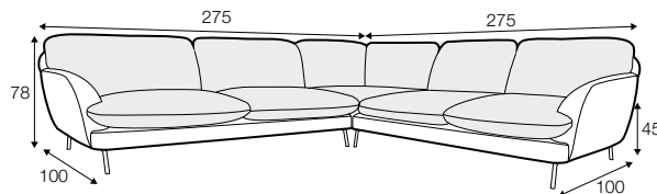
set 3
